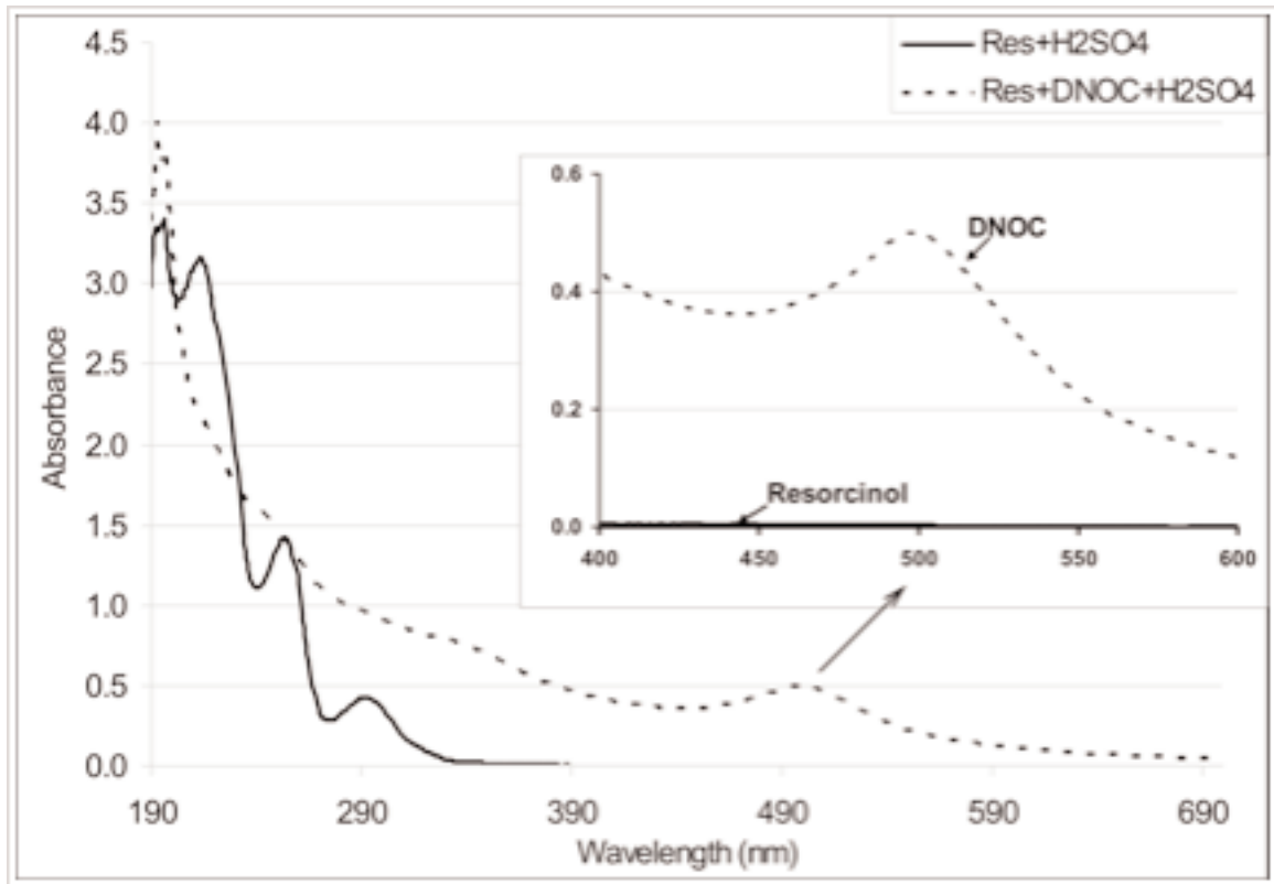
Figure 2 : Courbe du Résorcinol et du DNOC traité avec le résorcinol en UV visible
