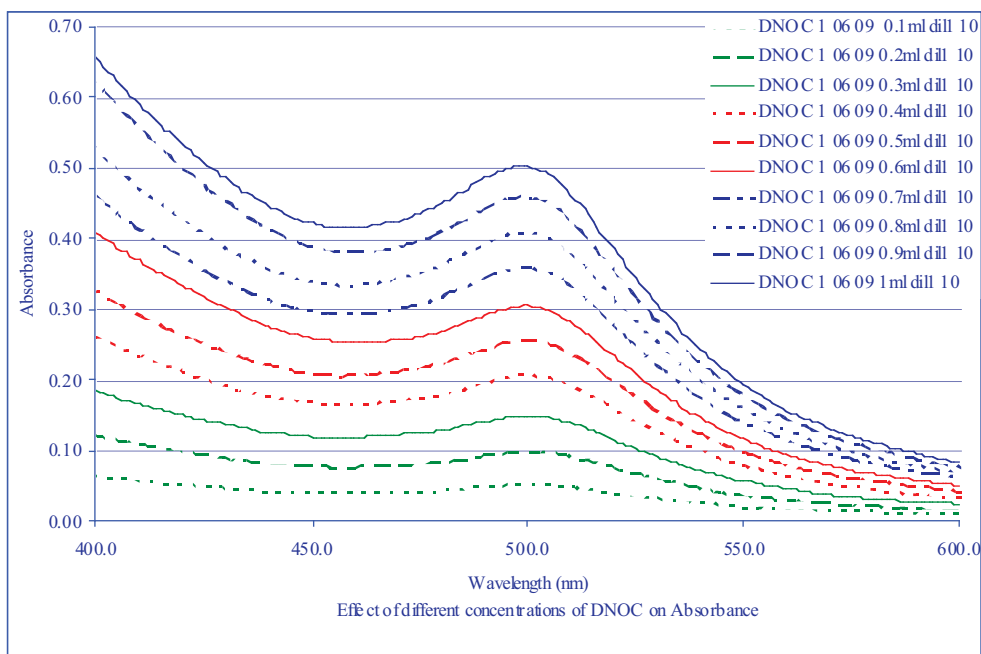
Figure 3 : Effet de différentes concentrations de DNOC sur l'absorbance de la solution colorée
