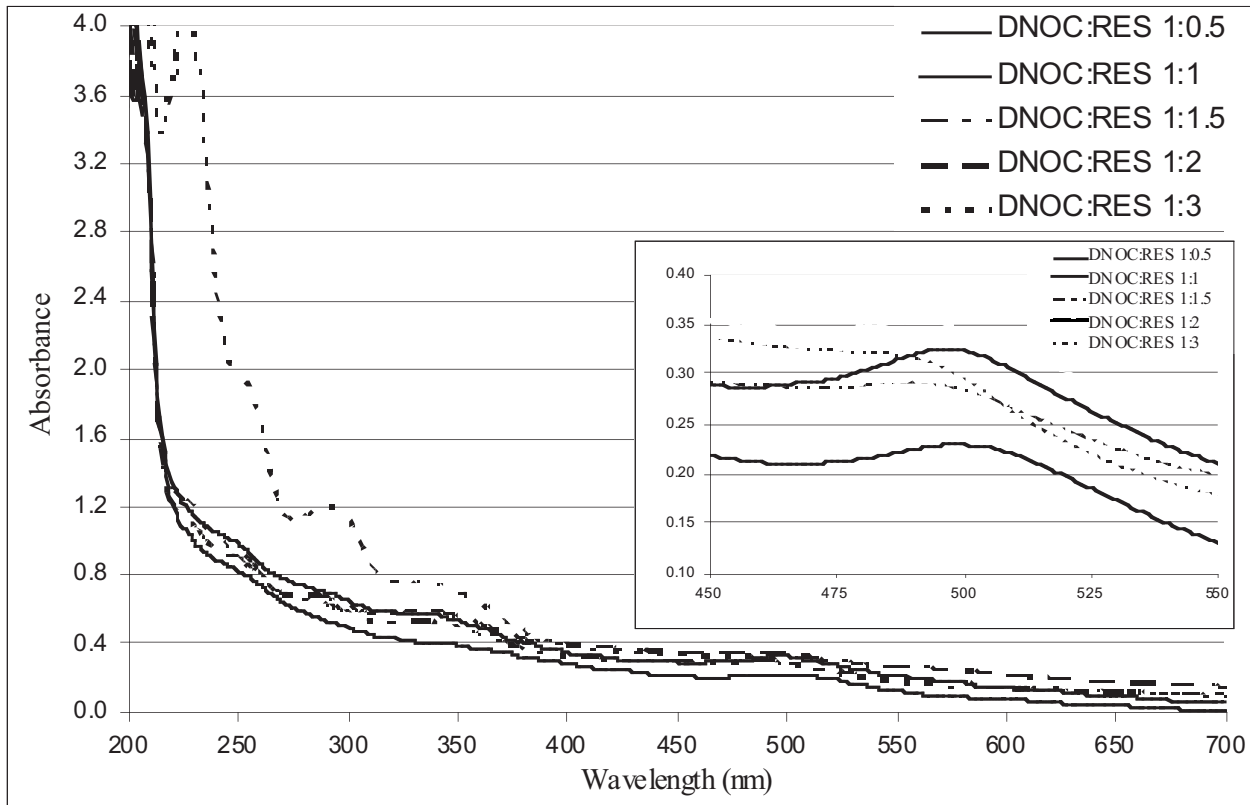
Figure 5 : Effet de différents ratios de concentrations molaires de DNOC: Résorcinol sur les absorbances des solutions colorées obtenues
