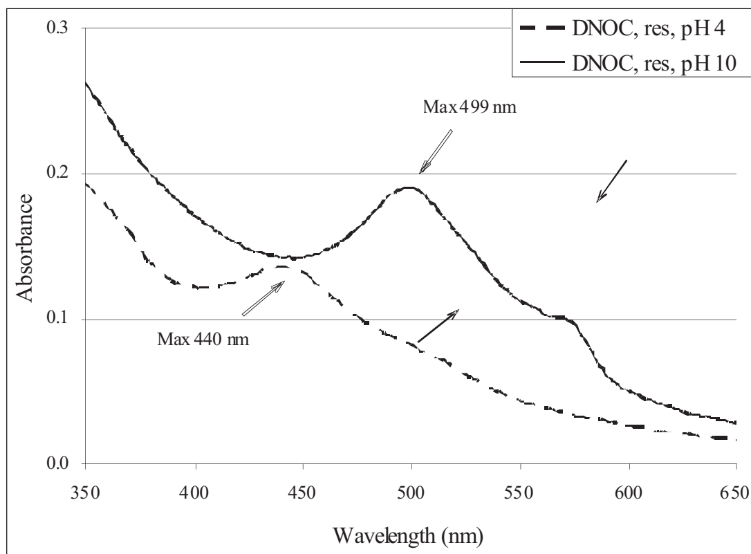
Figure 6 : Effet du pH sur l'absorbance du composé obtenu dans la réaction du résorcinol (res) avec le DNOC
